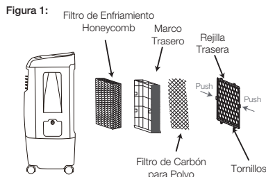
Figura 1: Extracción del filtro* de carbón para polvo / filtro de enfriamiento Honeycomb:
